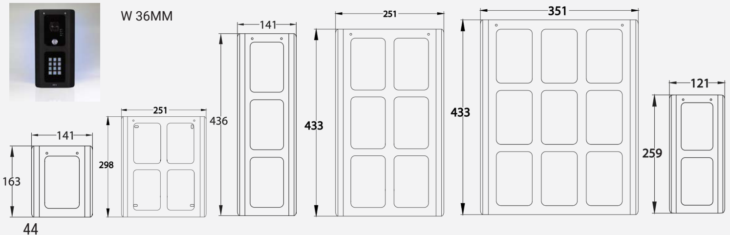
MOD-AB-1x1
